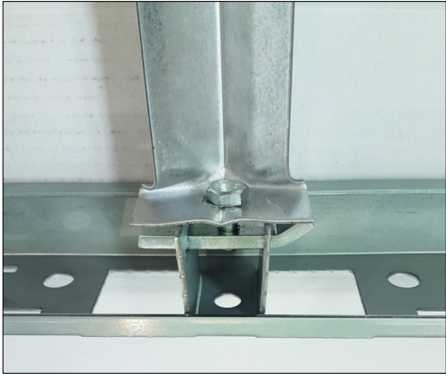
FOTO PARTICOLARE CAVALLOTTO E TIRANTE PHOTOS DETAIL CAVALLOTTO AND TIE
